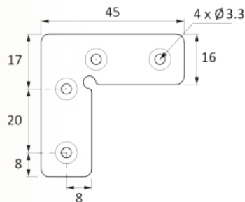
AH-21 Siku Frame Aluminium Untuk FA-21, FHD-21, FHD-23 Material : Besi Plat
