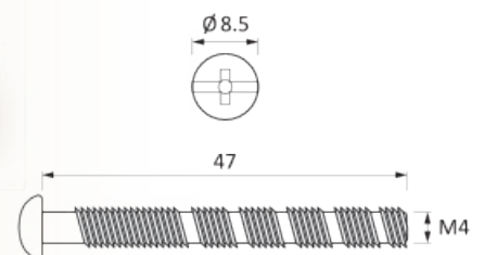
BOS-447 Skrup Patah-patah Ukuran Ø: M4 x 47 mm
