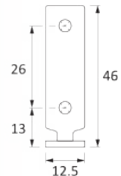
AH-56 Siku Frame Aluminium Untuk GP-56 & GP-72 Material : Besi Plat
