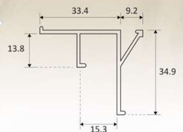
AS-99-B (Rel Bawah)
