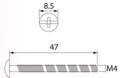
BOS-447 Skrup Patah-patah Ukuran Ø: M4 x 47 mm
