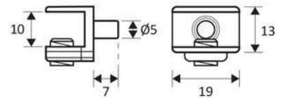
AKZ-14 Ambalan Kaca Zinc Material : Zinc Alloy Finish : Nickel
