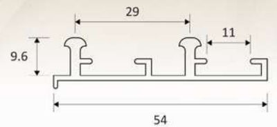
AS-99-A (Rel Atas)
