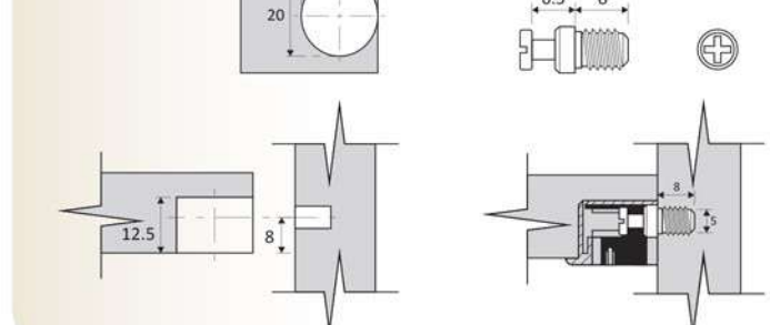
Fisher FIS-59 5 x 9 mm (Merah) FIS-512 5 x 12 mm (Putih) Pasangan Skrup : KSF-5533-9 KSF-6536-11
