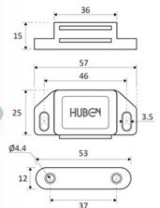
MP-46 Magnet Persegi Besar
