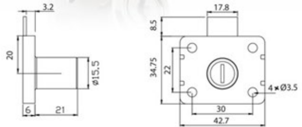
HUBEN HL-303 Kunci Laci
