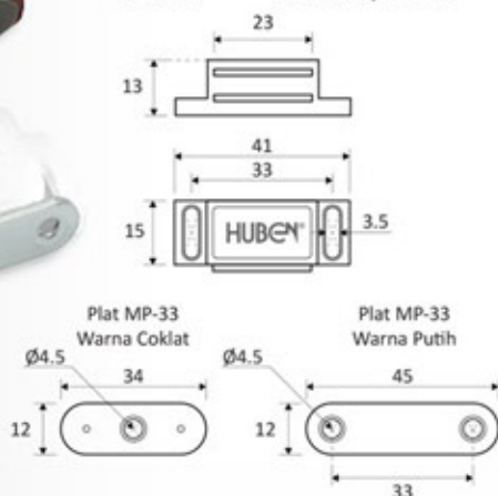
MP-33 Magnet Persegi
