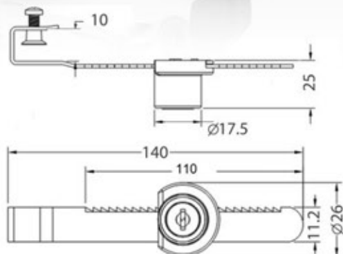
LENAGA LE-135 Kunci Gergaji
